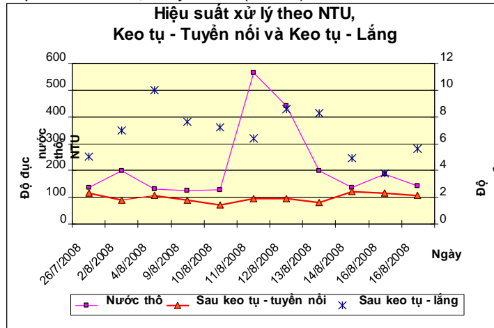
Hình 3. Thí nghiệm xử lý nước bằng công nghệ tuyển nổi, so sánh với keo tụ - lắng
