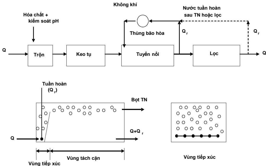
Hình 1. (Trên) Sơ đồ công nghệ xử lý nước với tuyển nổi áp lực; (Dưới) Bể tuyển nổi với vùng tiếp xúc và vùng tách chất rắn (Edzwald, 2007).
