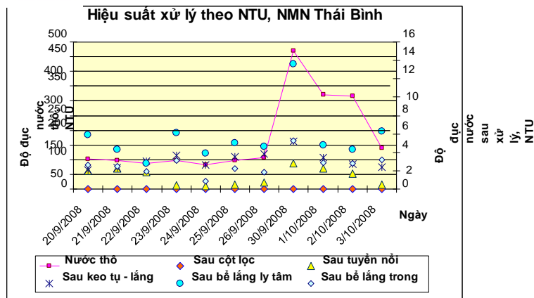
Hình 6. Kết quả thí nghiệm tại Nhà máy nước Thái Bình
