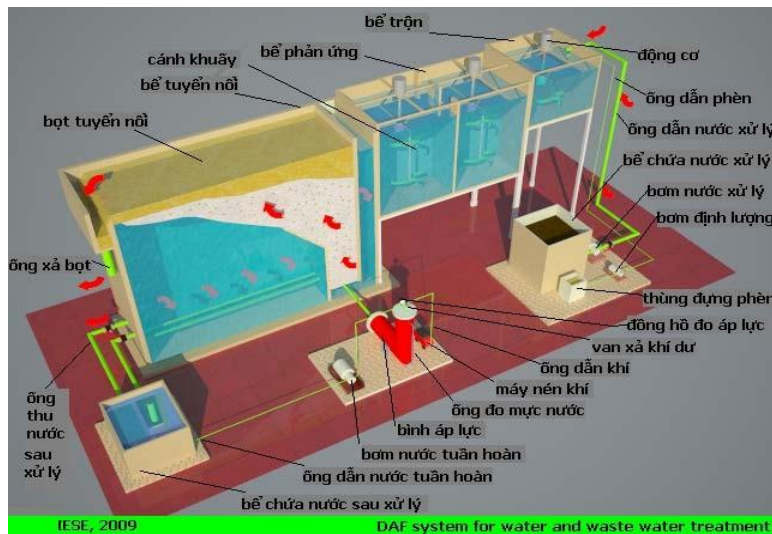
Hình 2. Sơ đồ hệ thống tuyển nổi áp lực pilot sử dụng trong nghiên cứu
